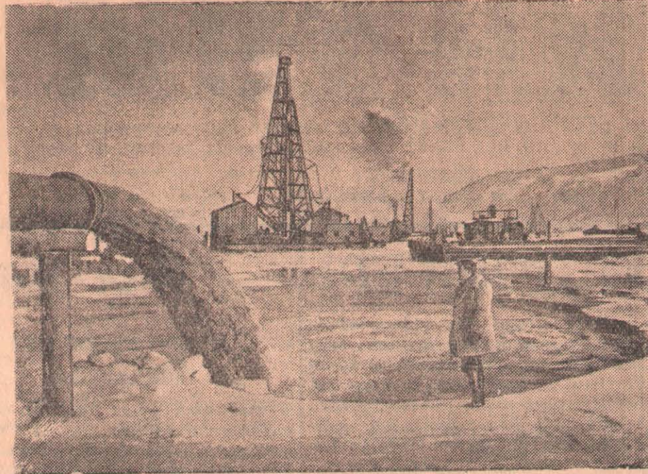
Куйбышев су электр станциясының құрылысы. Жигуди тауының етегіне құрылыстың шешуші участогі орналасқан. Қысқа уақыт ішінде мұнда дүние жүзіндегі ең ірі су электр станциясының үлкен котлованын көктемде Еділ суынан қоршайтын бөгет салынады. СУРЕТТЕ: котлован ішін суға толтыру. (СОТА-ның фотохроникасы).
