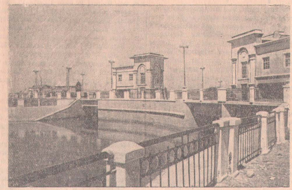
Ставрополь өлкесі. Кубань —Егорлыкск суландыру жүйесінің бас шлюзінің қуатты темір-бетон жабдықтары 54 километрлік канал бойынша өлкенің қуаң аудандарына Кубаньның суын жіберіп тұрады. СУРЕТТЕ: Кубань — Егорлыкск суландыру жүйесінің бас шлюзінің көрінісі.
