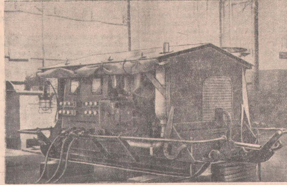
ССРО Совхоздар министрлігінің Ростов механика зауыды жылжымалы «ПЭС—8» электр станциясын жасап шығарды. Станцияның көлемі кішкентай, ауырлығы 820 килограмм. Станция генераторының қуаттылығы 8 киловатт, оны 13 аттың күші бар дизель моторы қозғалтып тұрады.
