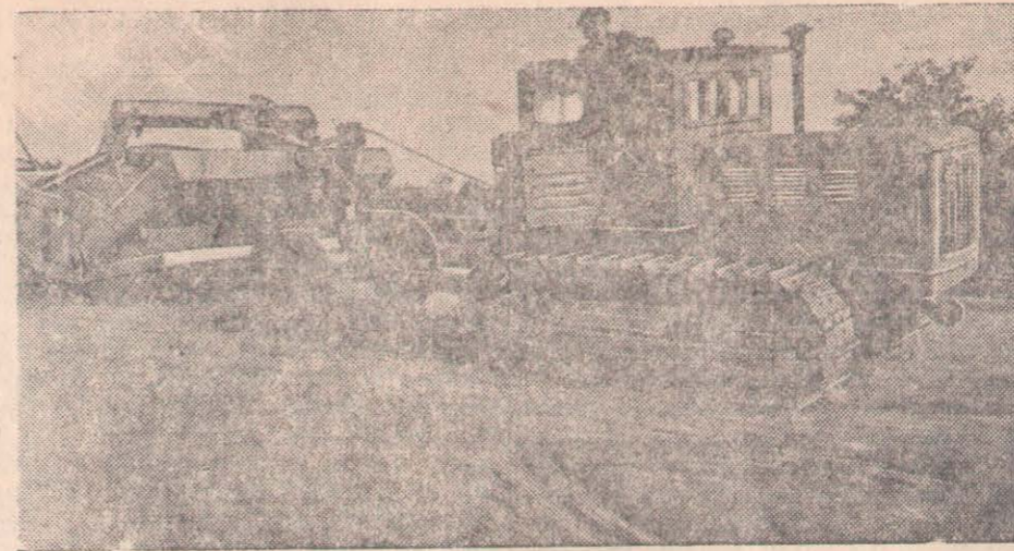
Петропавл машина-жол станциясына жаңа техника үздіксіз келуде. Станция жақында екі скрепер мен екі бульдозер алды. СУРЕТТЕ: жаңадан алынған скрепер. Суретті түсірген А. Розенштейн.
