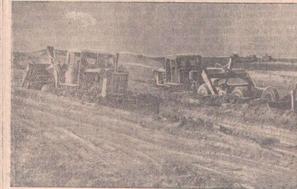
Біздің Республикамыздағы ең ірі Арыс-Түркістан каналы құрылысының жұмыс қарқыны күн санап арта түсуде. СҮРЕТТЕ: Бұғын су қоймасы плотинасының құрылысында жұмыс істейтін скреперлер мен бульдозерлер. (ҚазТАГ-тың фотохроникасы).
