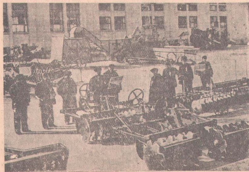
На снимке: на открытой площадке выставки. Сельскохозяйственные машины, изготовленные в Китае. Фото Люй Ху-миня. Агентство Синьхуа.
