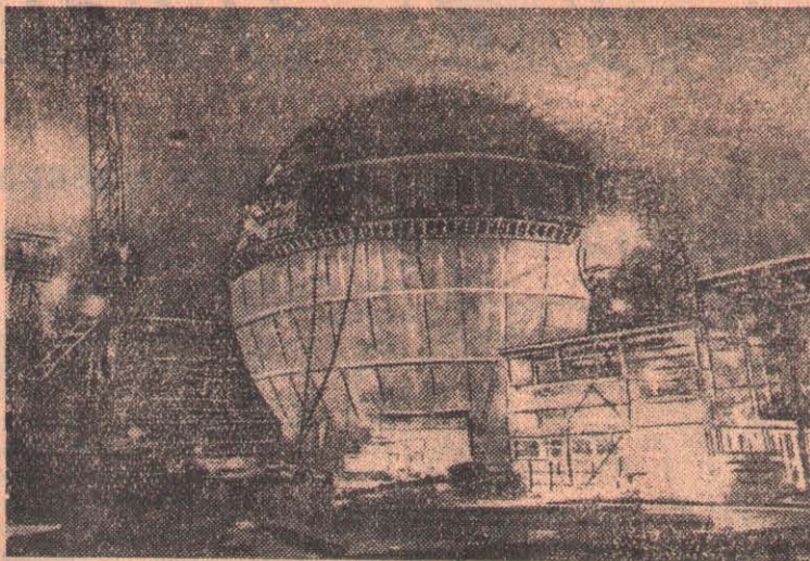
Англия. На строительстве атомного реактора в научно-исследовательском центре в Даунри (Шотландия). Диаметр этого герметически закрытого шара, в котором разместится реактор, превышает диаметр купола знаменитого собора святого Павла в Лондоне.
